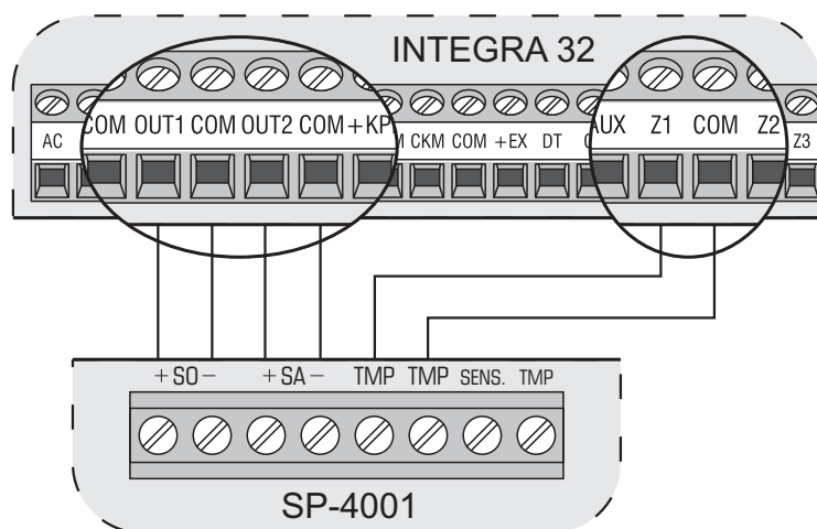
Рис. 20. Способ подключения оповещателя без собственного питания к силовым выходам (на примере SP-4001 и ПКП INTEGRA 32). Выход OUT1 управляет оптической сигнализацией, а выход OUT2 – акустической (силовой выход с нормальной поляризацией – включение осуществляется подачей напряжения +12 В). Зона Z1 запрограммирована как саботажная (шлейф типа NC, тип реакции 9. 24ч САБОТАЖНАЯ).
