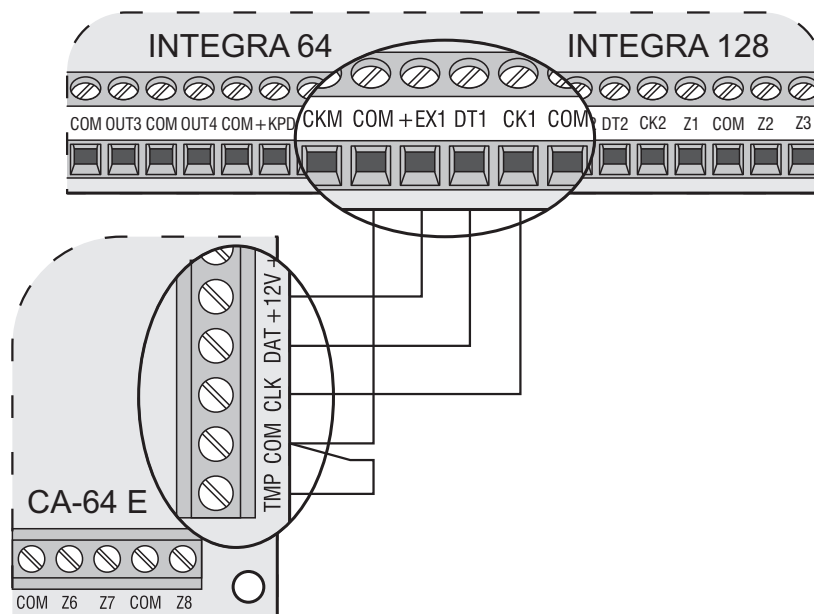
Рис. 11. Способ подключения модуля расширения без блока питания на примере модуля расширения зон CA-64 E и ПКП INTEGRA 64/INTEGRA 128. Модуль расширения установлен в один корпус вместе с ПКП, поэтому клемма TMP замкнута на COM (массу).
