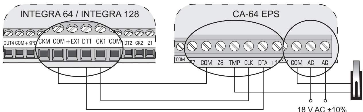
Рис. 12. Способ подключения модуля расширения с блоком питания на примере модуля расширения зон CA-64 EPS и ПКП INTEGRA 64 / INTEGRA 128. К клеммам TMP и COM подключен тамперный контакт корпуса. Клеммы AC подключите к клеммам вторичной обмотки сетевого трансформатора.
