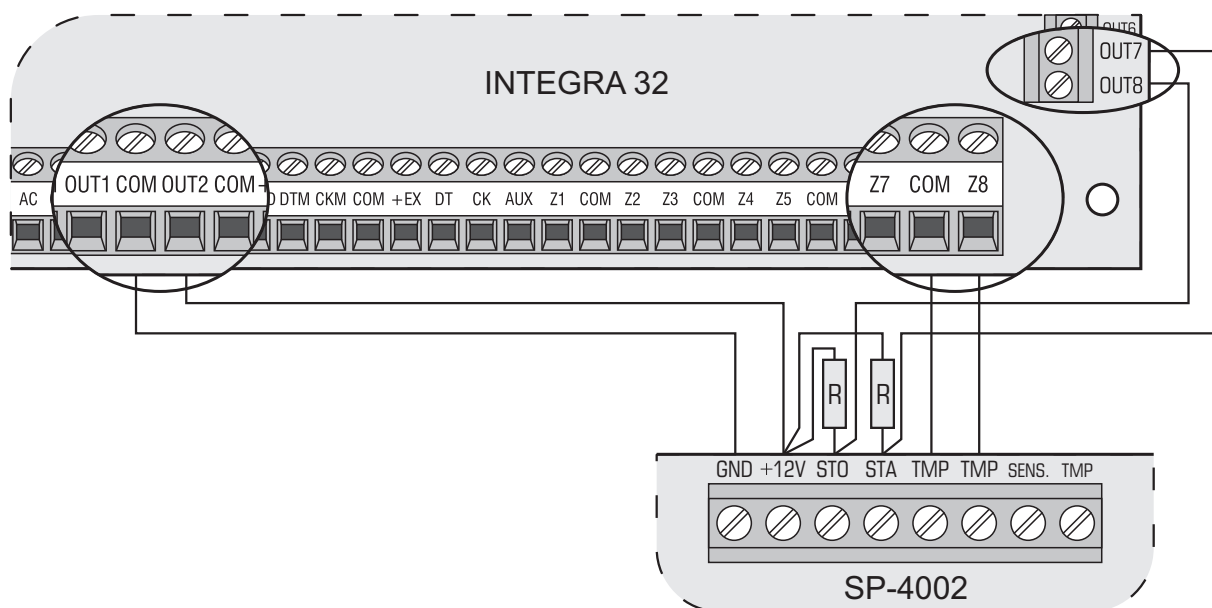
Рис. 21. Способ подключения оповещателя с собственным питанием к выходам ПКП (на примере SP-4002 и ПКП INTEGRA 32). Силовой выход OUT2 запрограммирован как выход питания. Выход OUT7 управляет акустической сигнализацией, а выход OUT8 – оптической (слаботочные выходы с нормальной поляризацией – включение осуществляется замыканием на массу). Зона Z8 запрограммирована как саботажная (шлейф типа NC, тип реакции 9. 24ч САБОТАЖНАЯ). Величина номинала резисторов R – 2,2 кΩ.
